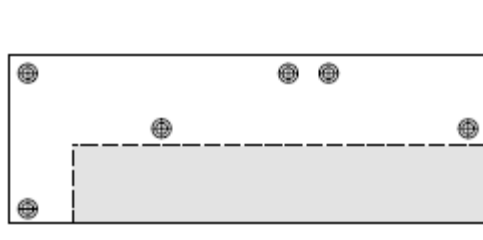
Aangezicht morteldrager bijv. Cempanel Met overlaping van het zonnescerm
